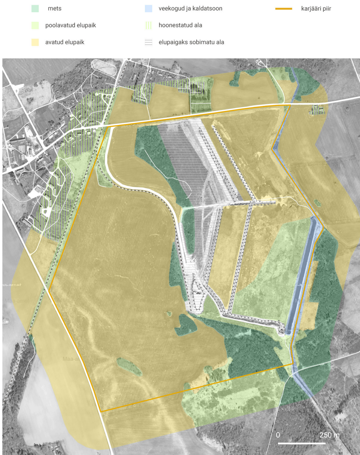
Pilt 19. Ubja põlevkivikarjääri imetajate elupaigad. Figure 19. Habitats of mammals at Ubja oil shale quarry.
