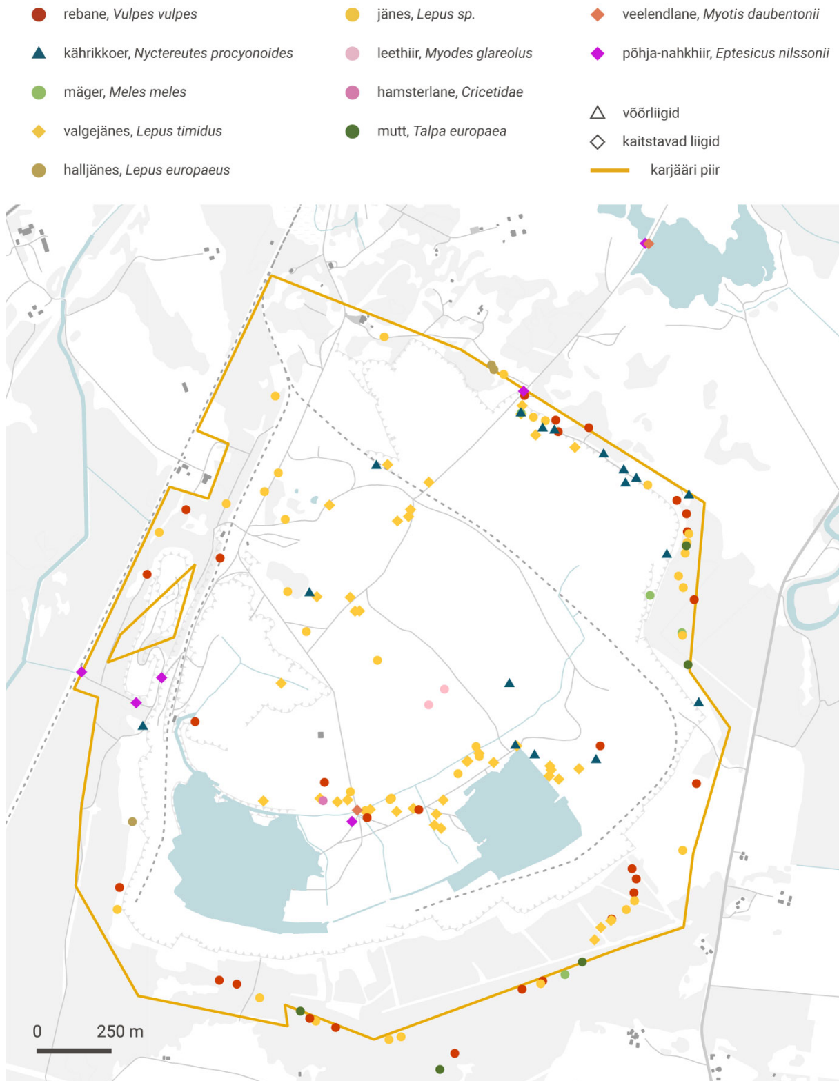
Pilt 16. Aru-Lõuna lubjakivikarjääris välitööl registreeritud väike- ja pisiimetajate ning nende tegevusjälgede vaatluskohad.
