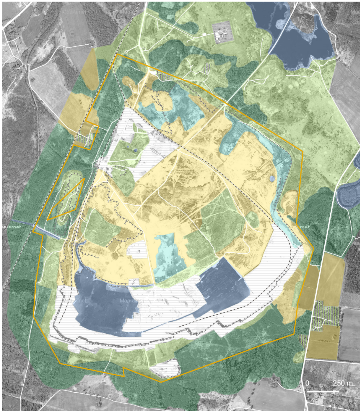
Pilt 12. Aru-Lõuna lubjakivikarjääri imetajate elupaigad.
